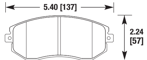
SUBARU, SCION
