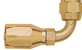
90° S.A.E. 37° SWIVEL
